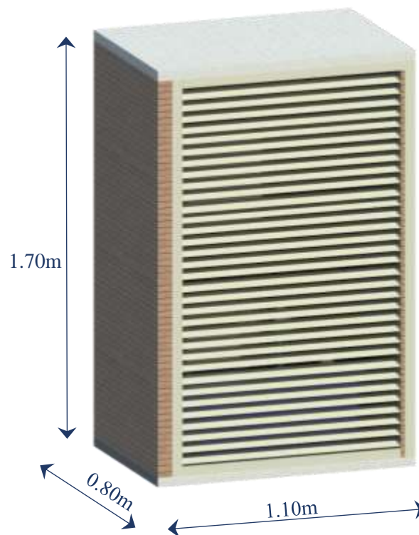
Dimensiones interiores de gabinete
