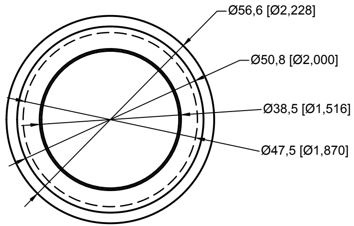
VISTA SUPERIOR
