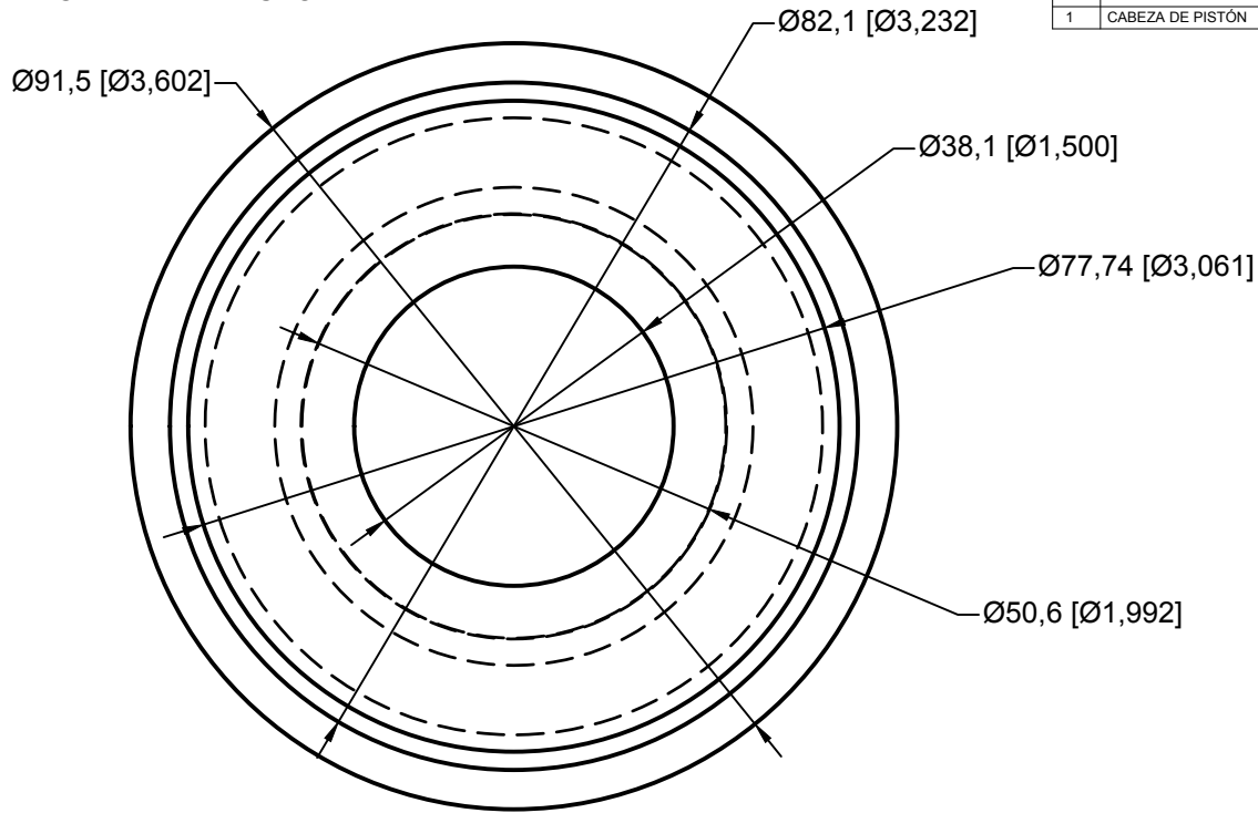
VISTA SUPERIOR
