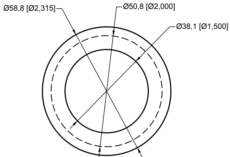
VISTA SUPERIOR
