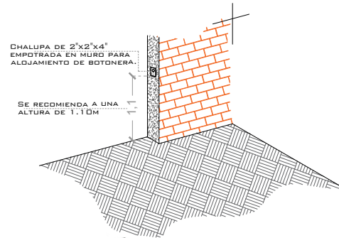
CHALUPA DE 2'x2'x4' EMPOTRADA EN MURO PARA ALOJAMIENTO DE BOTONERA.
