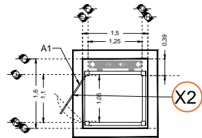
DIMENSIONES DE CABINA
