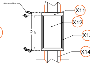
DIMENSIONES DE CABINA (ALTURAS)
