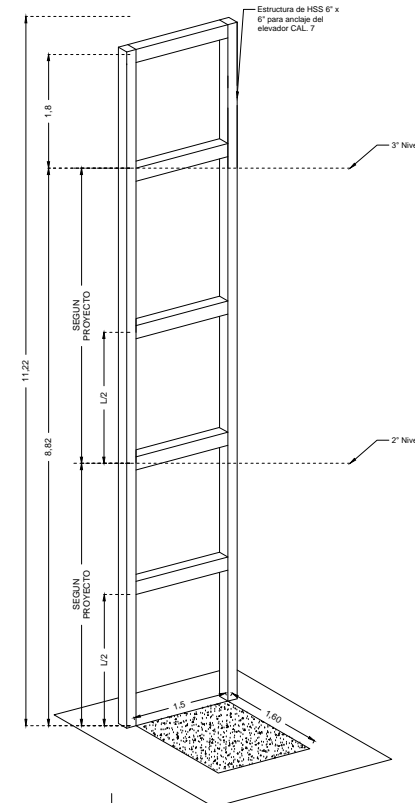
REQUERIMIENTOS DE REFUERZO (ESTRUCTURA)
