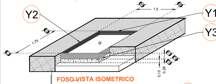
FOSO-VISTA ISOMETRICO
