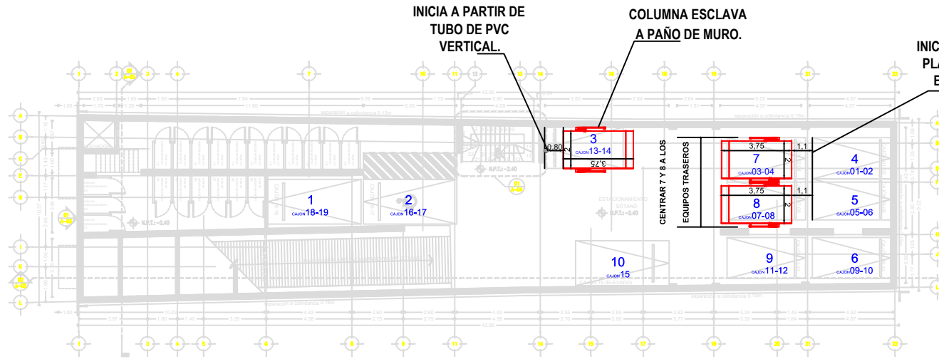
PLANTA SOTANO -2.40
