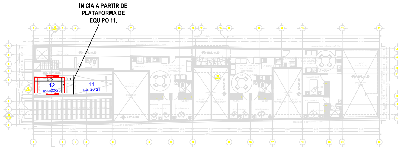
PLANTA BAJA +1.80
