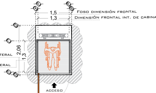
ELEVADOR SEMICOMPLETA PLANTA
