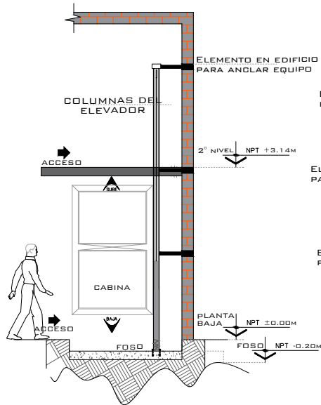
ELEVADOR SEMICOMPLETA LATERAL
