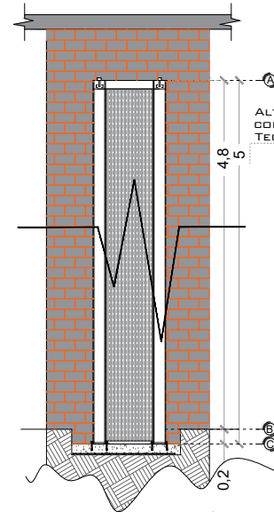
ALTURA DE MECANISMO TECNORAMPA
