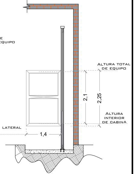
ALTURA DE CABINA SEMICOMPLETA
