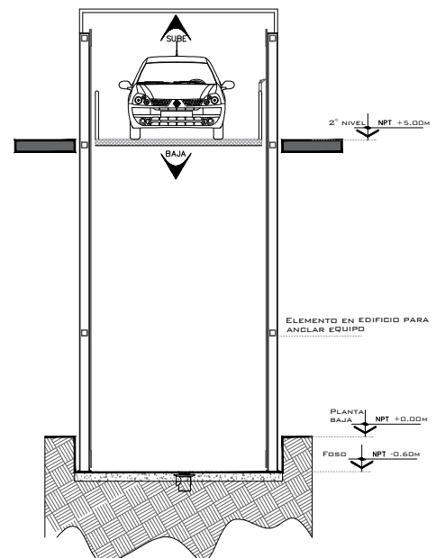
ELEVADOR DE AUTOS FRONTAL
