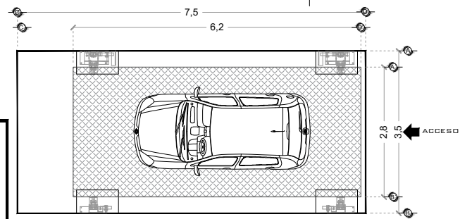
ELEVADOR DE AUTOS PLANTA
