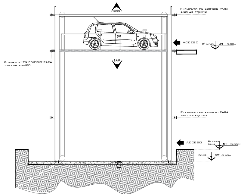
ELEVADOR DE AUTOS LATERAL
