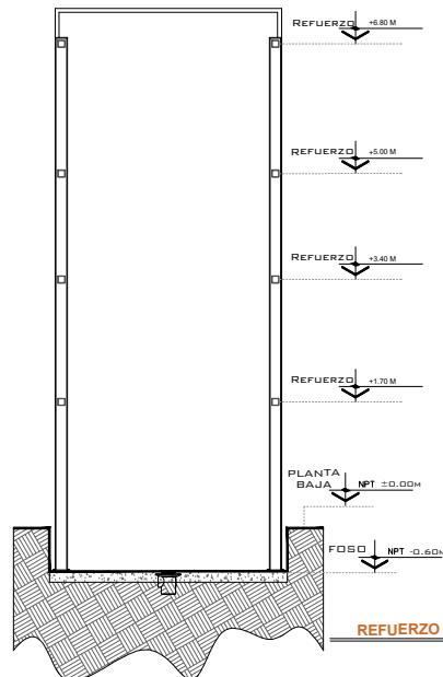
ALTURA DE COLUMNAS CARGA
