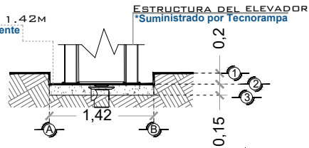
FOSO DEL ELEVADOR VISTA FRONTAL
