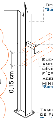
COLUMNA DEL ELEVADOR ISOMETRICO
