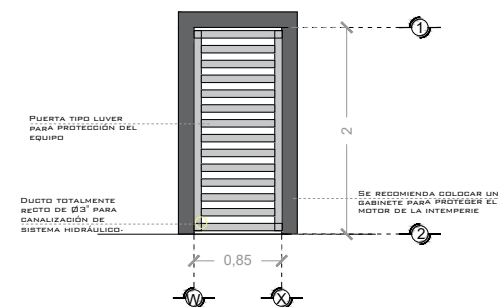
DESCRIPCIÓN DE UNIDAD HIDRÁULICA GABINETE (VISTA FRONTAL)
