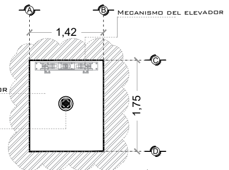
FOSO DEL ELEVADOR VISTA PLANTA
