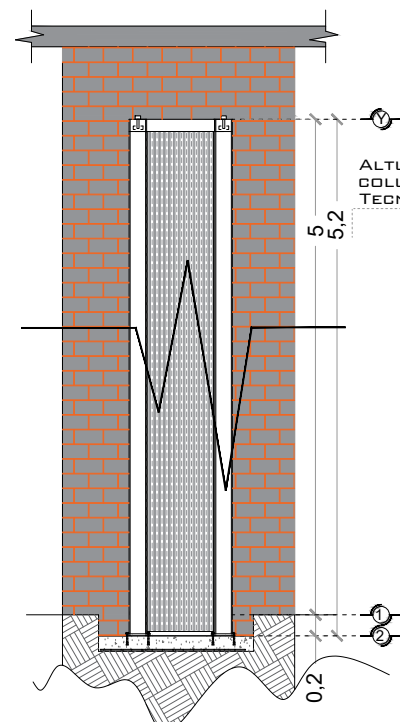
ALTURA DE MECANISMO TECNORAMPA
