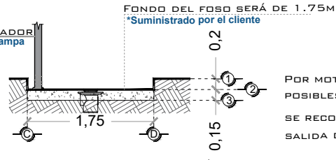
FOSO DEL ELEVADOR VISTA LATERAL
