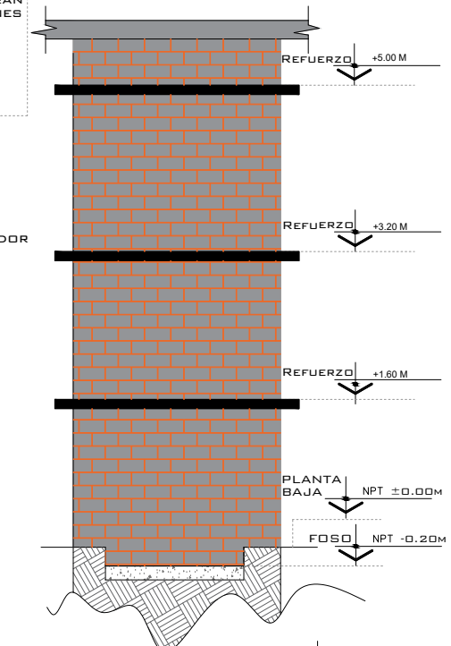
REFUERZO DE ANCLAJE ALTURAS
