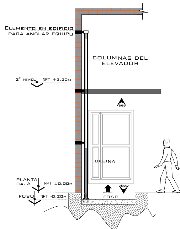
ELEVADOR SEMICOMPLETA LATERAL
