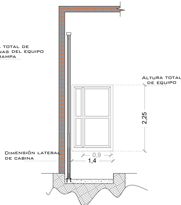
ALTURA DE CABINA SEMICOMPLETA
