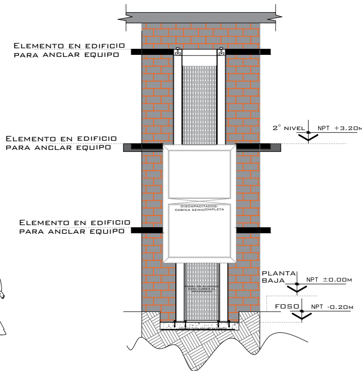
ELEVADOR SEMICOMPLETA FRONTAL
