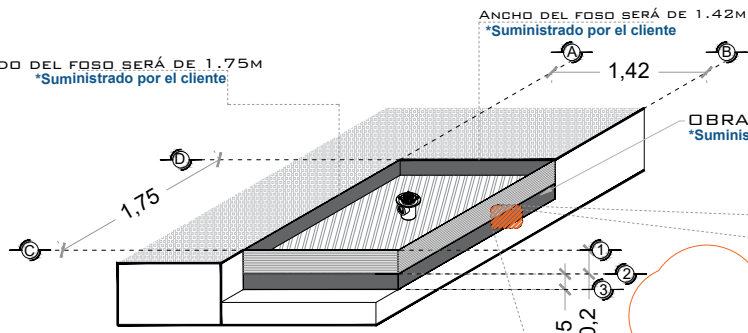
FOSO DEL ELEVADOR ISOMETRICO
