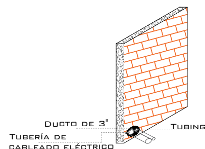
DUCTO DE ALIMENTACION ISOMETRICO
