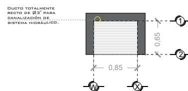
DESCRIPCIÓN DE UNIDAD HIDRÁULICA GABINETE (VISTA PLANTA)
