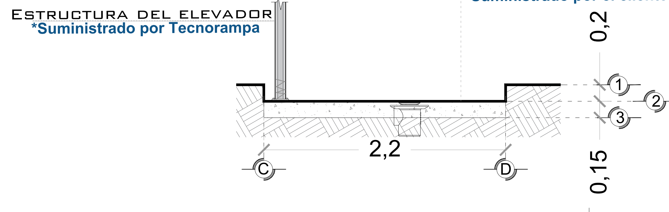
FOSO DEL ELEVADOR VISTA LATERAL
