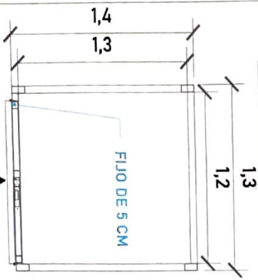
ACCESO PB-1ER NIVEL CABINA (VISTA EN PLANTA)
