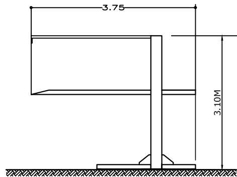
VISTA LATERAL
