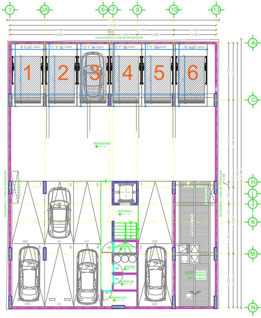
1 PLANTA SEMISOTANO NIVEL -1.35
