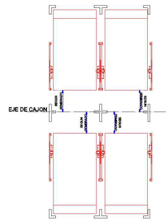
EJEMPLO DE DISTANCIA DE RESGUARDO PARA DOBLE BATERIA
