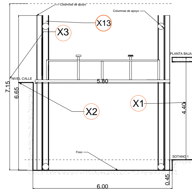
ALZADO (RECORRIDO)
