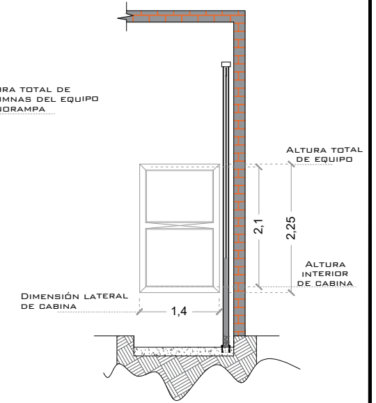
ALTURA DE CABINA SEMICOMPLETA
