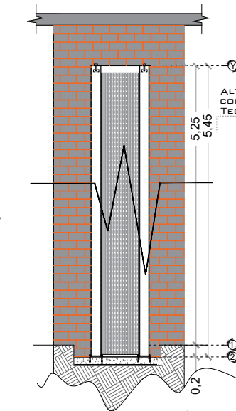
ALTURA DE MECANISMO TECNORAMPA
