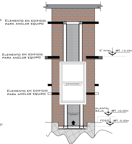
ELEVADOR SEMICOMPLETA FRONTAL
