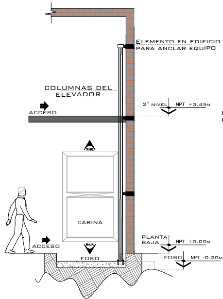
ELEVADOR SEMICOMPLETA LATERAL
