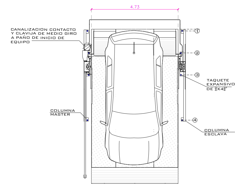
VISTA SUPERIOR
