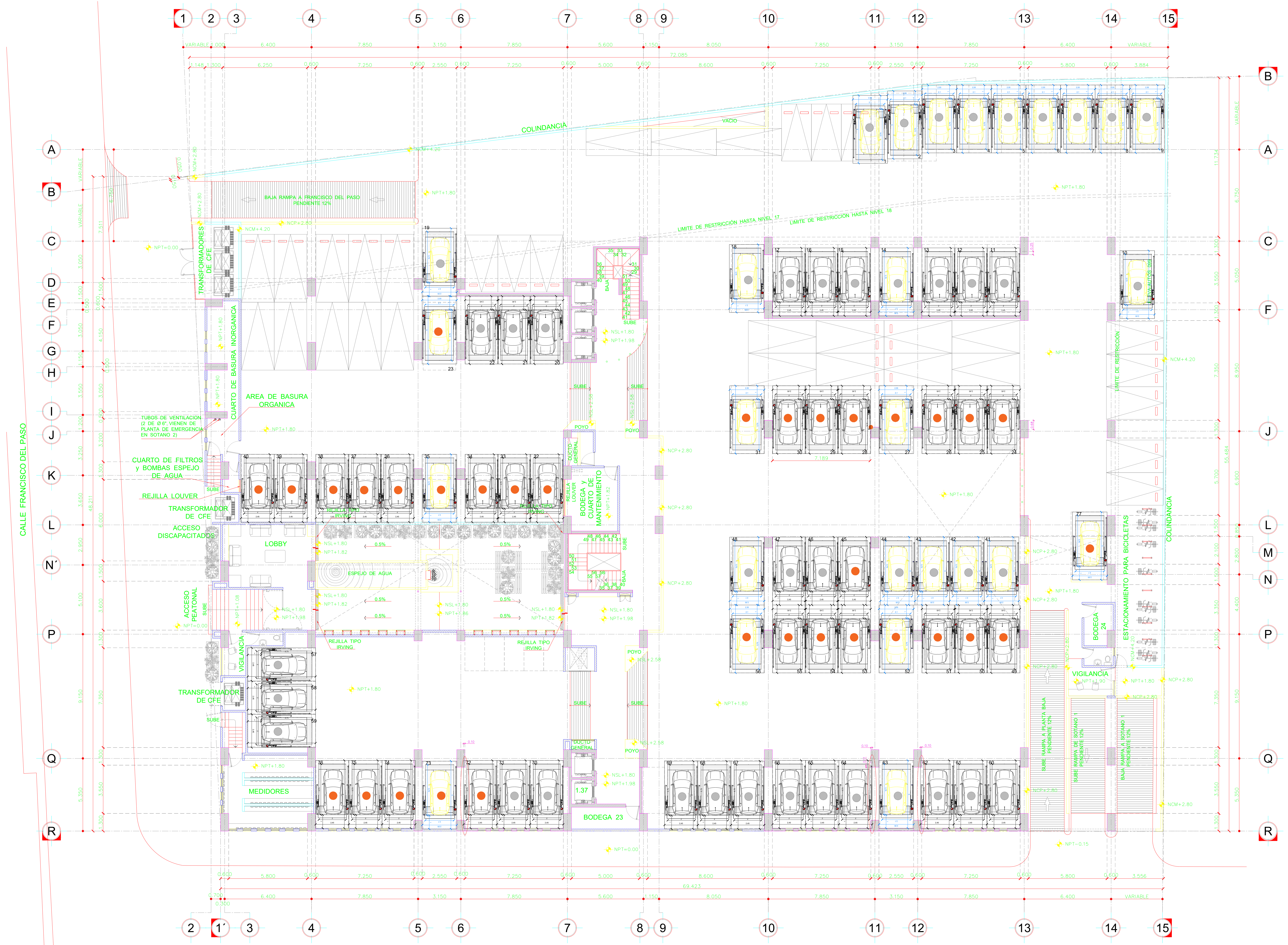
PLANTA BAJA
