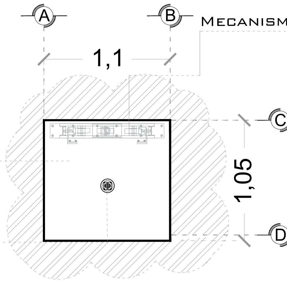
FIRME DE CONCRETO PARA ELEVADOR VISTA PLANTA
