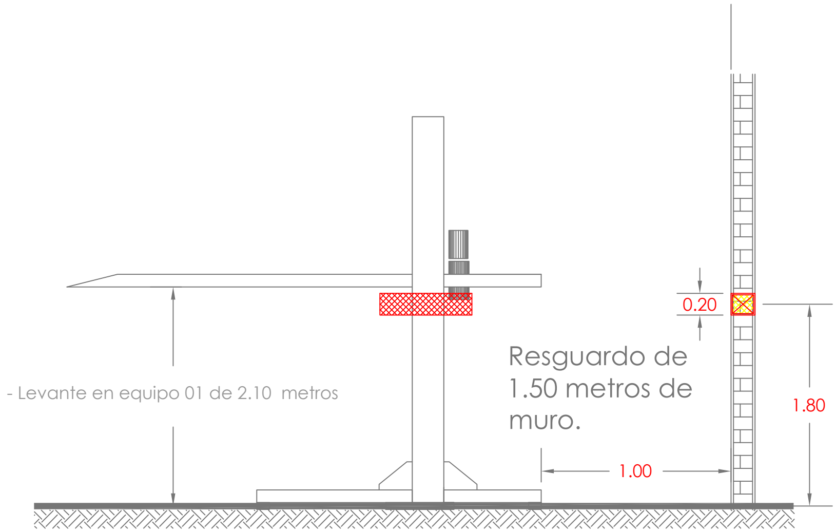
VISTA LATERAL croquis referencial tr one
