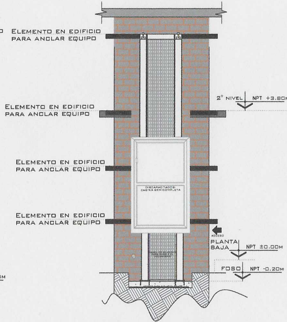
ELEVADOR SEMICOMPLETA FRONTAL
