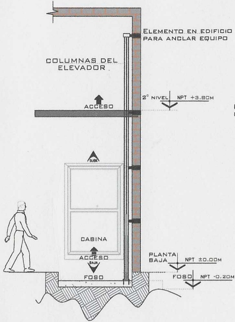
ELEVADOR SEMICOMPLETA LATERAL
