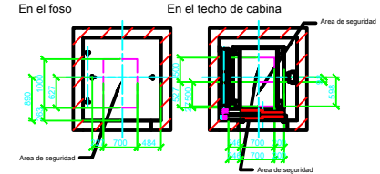
Situación del espacio de refugio 1:50
