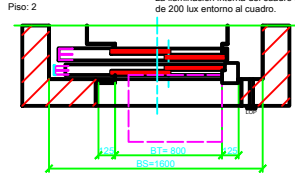
Detalle de puerta 1:20
