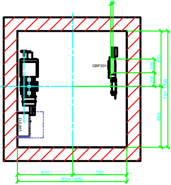
Techo del hueco 1:20
