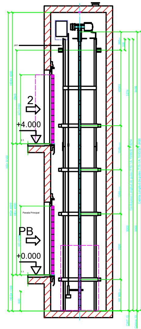
Sección A-A 1:25
