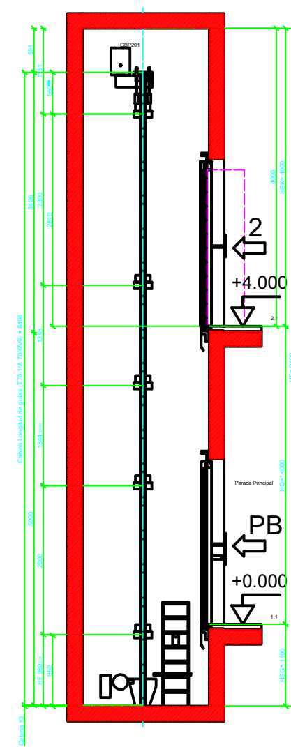
Sección B-B 1:25
