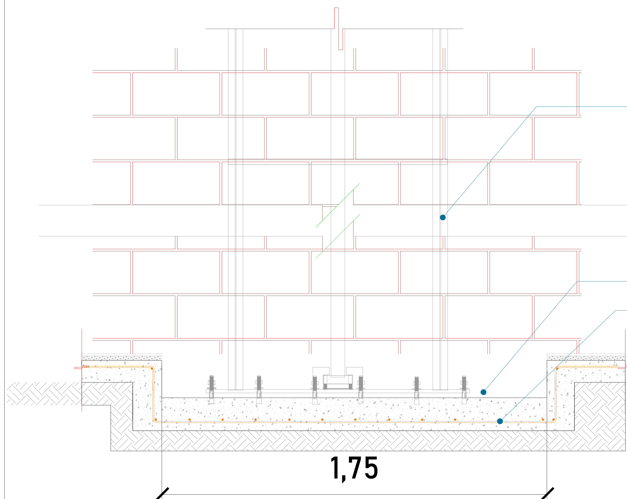
FOSO (VISTA FRONTAL) FOSO DE 35 cm
