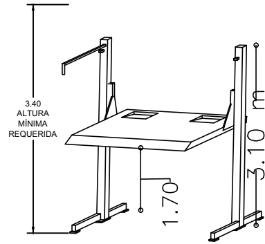
VISTA ISOMÉTRICO
