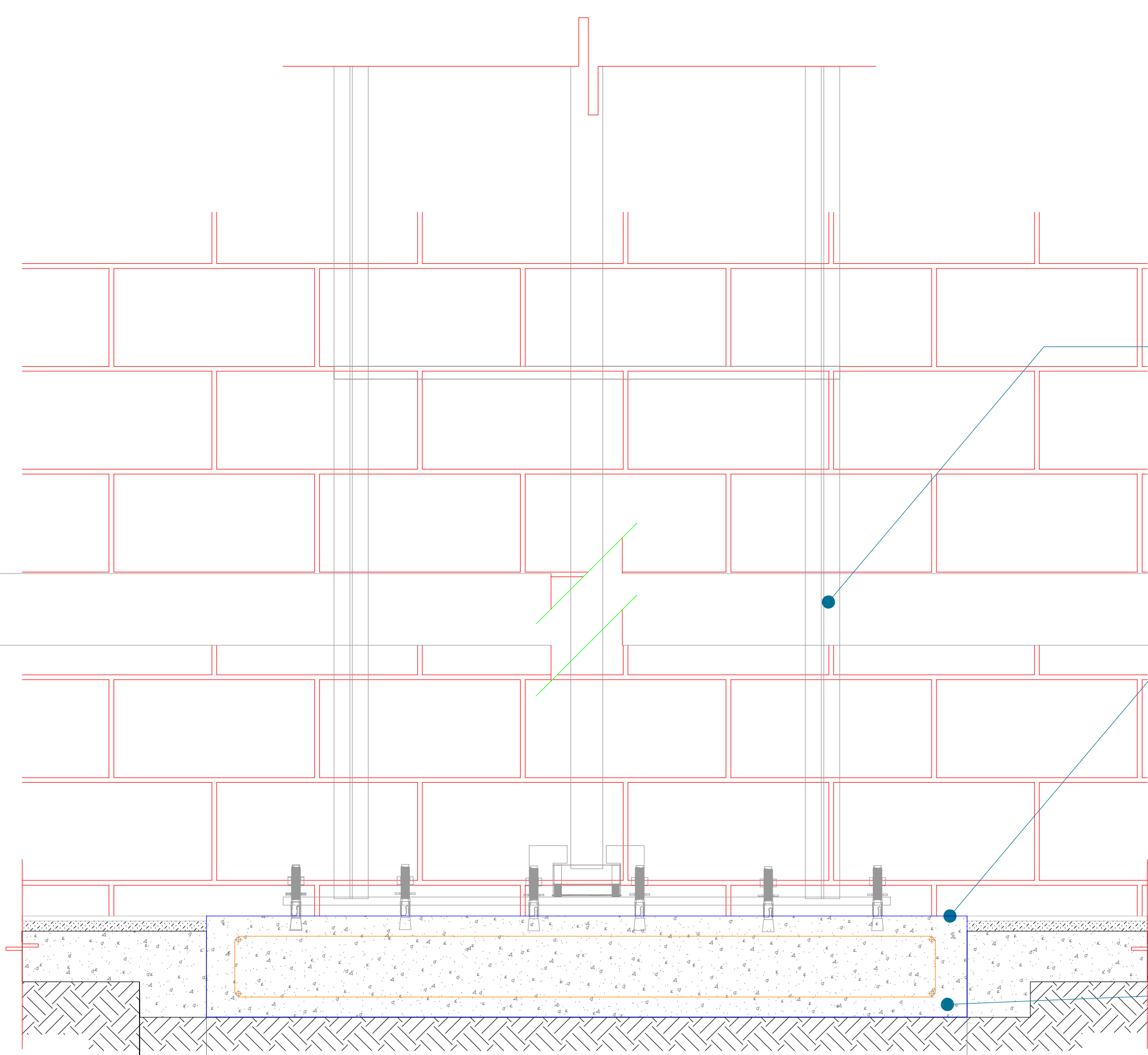
FOSO (VISTA FRONTAL)
