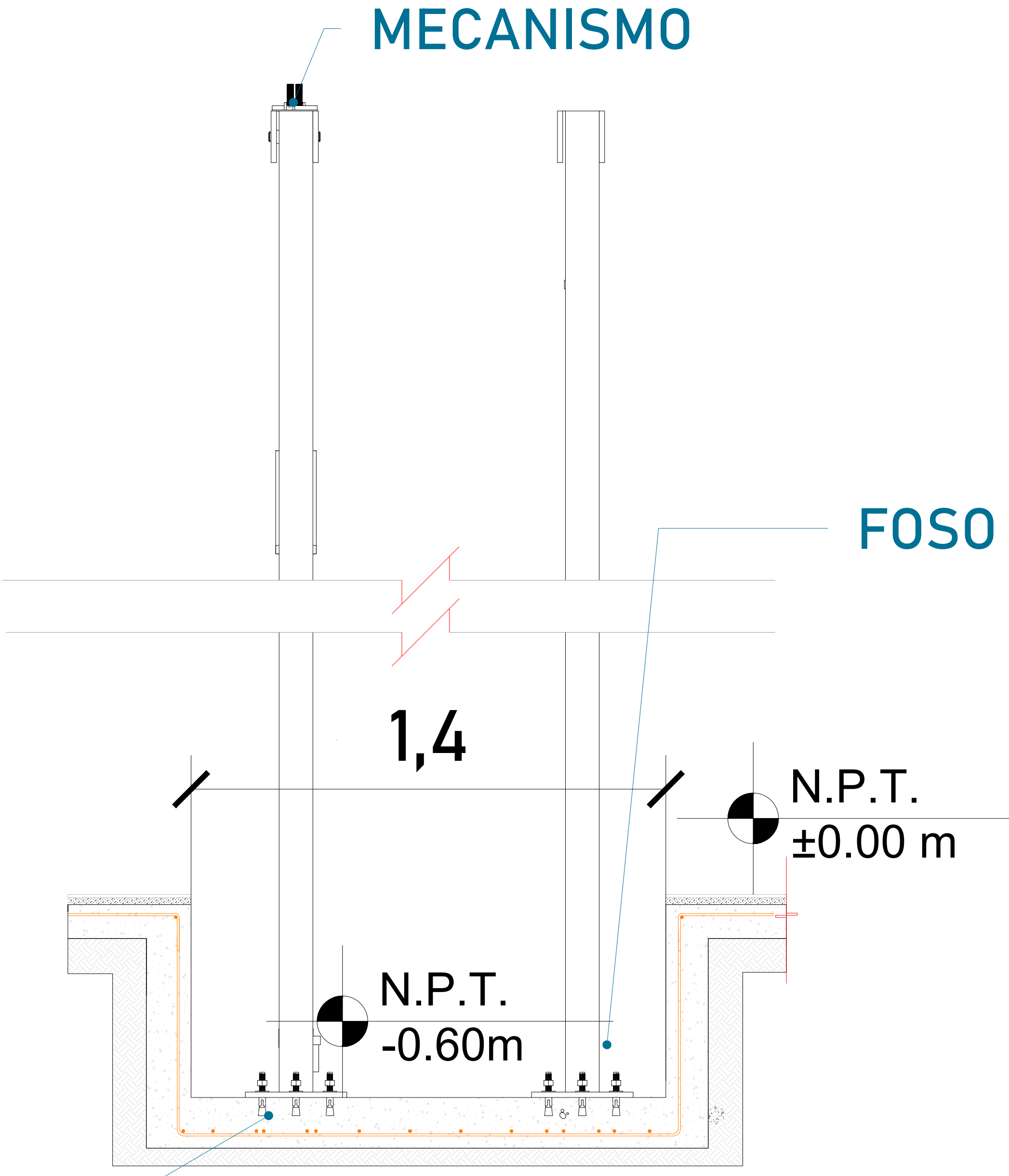
FOSO (VISTA FRONTAL)
