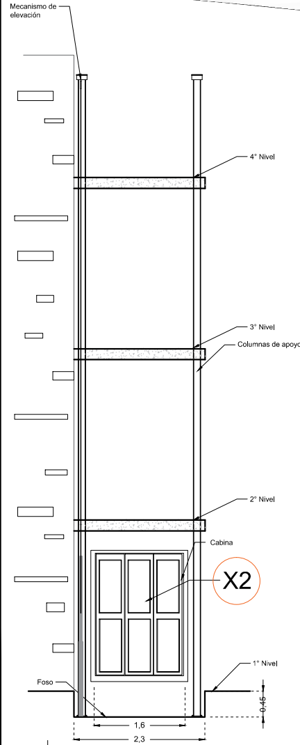
ALZADO (ESTRUCTURA)
