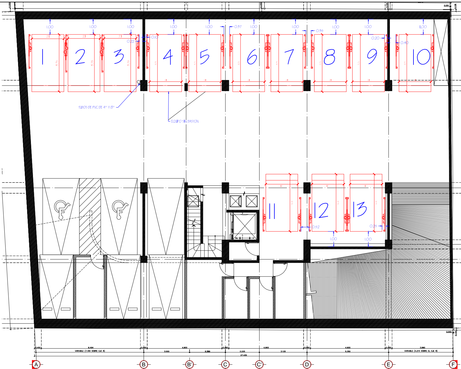
PLANTA SOTANO 2
