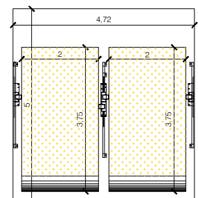
2 JUEGOS DE 2 RAMPAS EMPATADAS 2.00M X 3.75M
