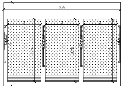
4 JUEGOS DE 3 RAMPAS EMPATADAS 2.00M X 3.75M
