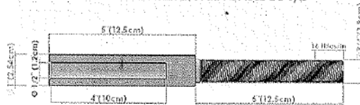
TERMINAL STANDAR PARA CABLE DE 1/2"
