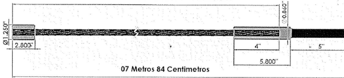
TOPE STANDAR PARA CABLE DE 1/2"
