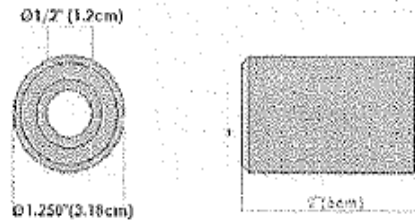
TOPE STANDAR PARA CABLE DE 1/2"
