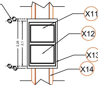
DIMENSIONES DE CABINA (ALTURAS)
