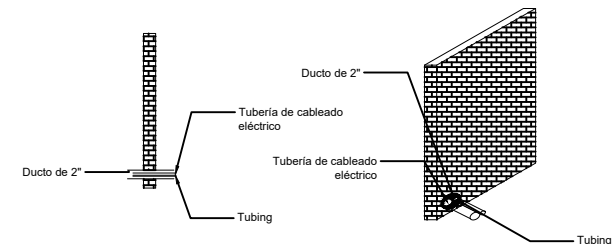
DUCTO DE 2" EN EL GABINETE
