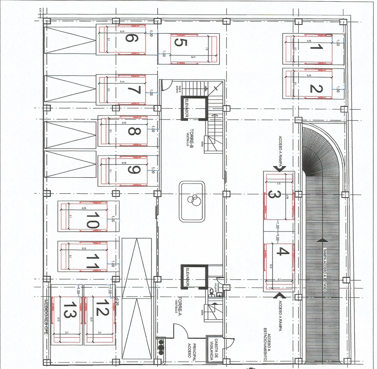
DETALLE DE LA INSTALACION DE LA RAMPAS EN UNO DE LOS ACCESOS A LA ESTACIONAMIENTO (CANTON)
