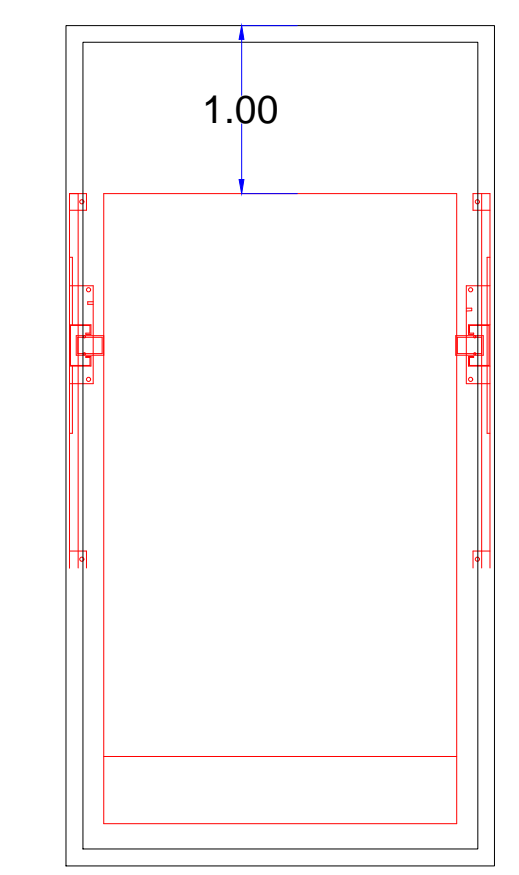
EJEMPLO DE INSTALACION DE RAMPAS EN LUGAR DE ESTACIONAMIENTO (RAMPA CENTRADA A CAJON AISLADO)
