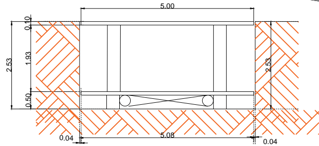
CORTE DE UNDER RAMP (Altura de foso 2.53 m)
