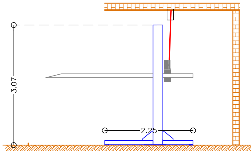
VISTA LATERAL
