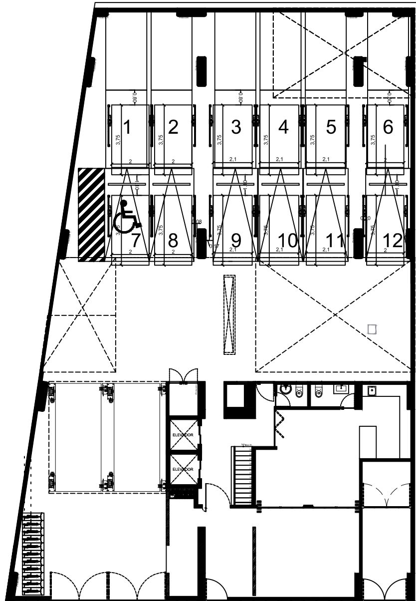
PLANTA BAJA
