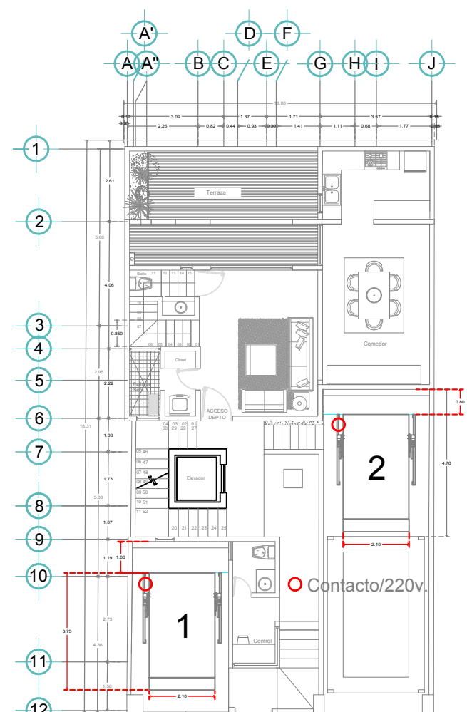
PLANTA BAJA
