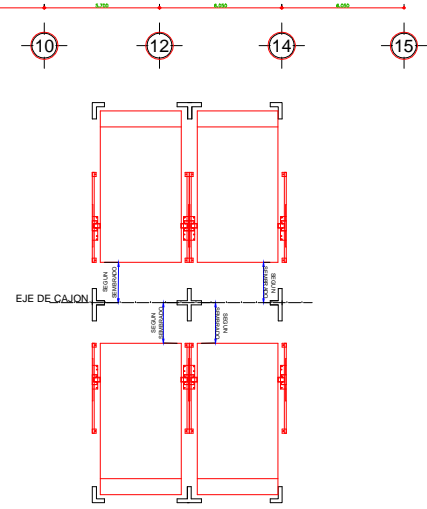
EJEMPLO DE DISTANCIA DE RESGUARDO PARA DOBLE BATERIA
