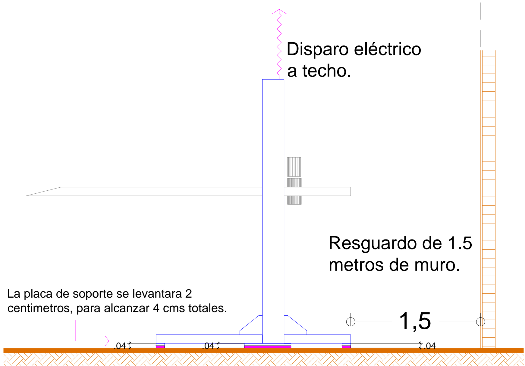
VISTA LATERAL
