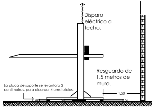
VISTA LATERAL
