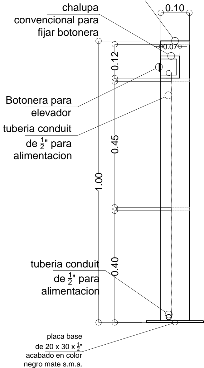
ALZADO LATERAL
