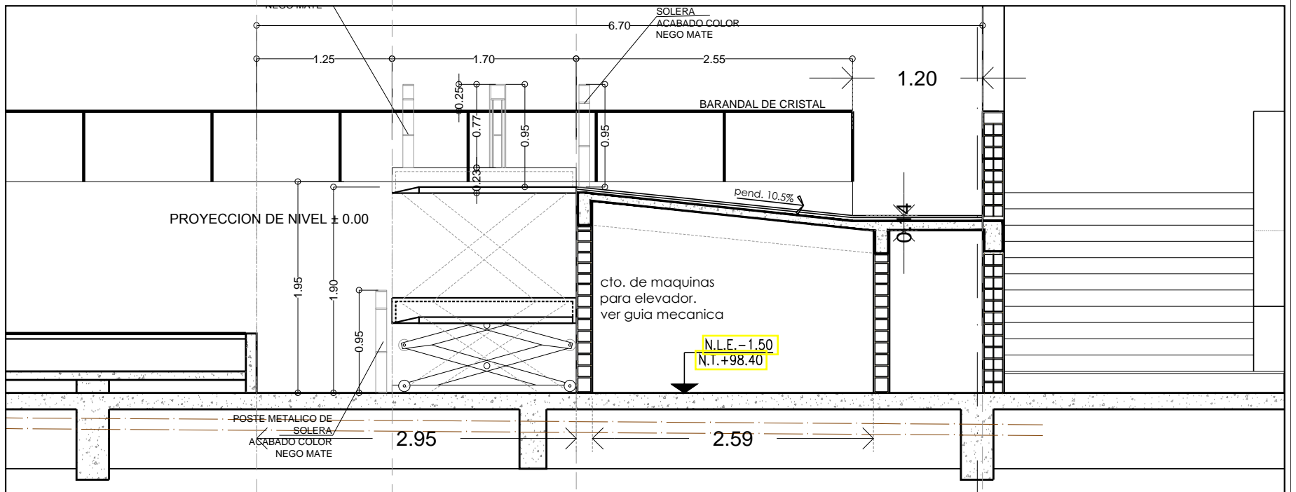
CORTE-A
