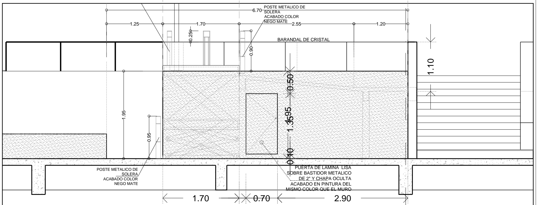
FACHADA-1
