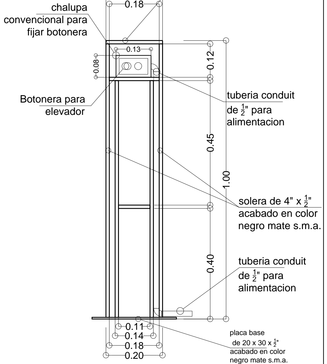
ALZADO FRONTAL
