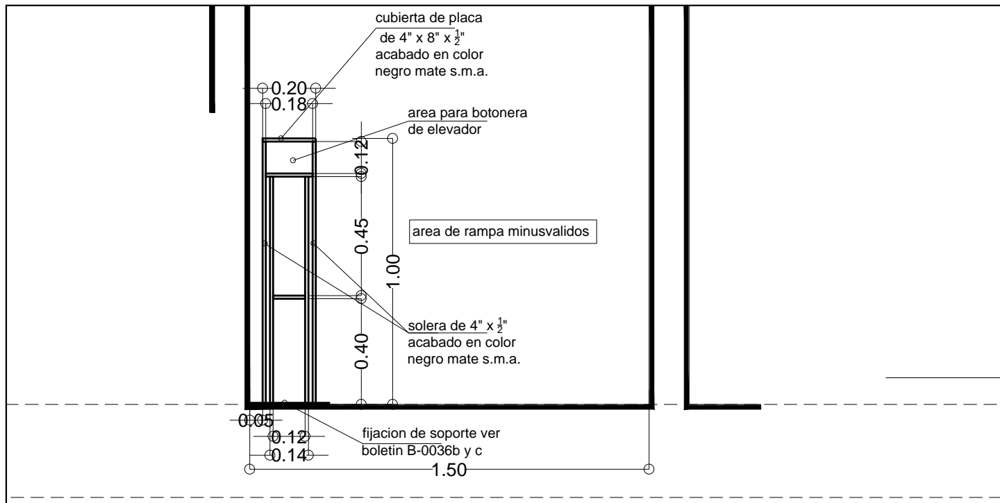
CORTE-C
