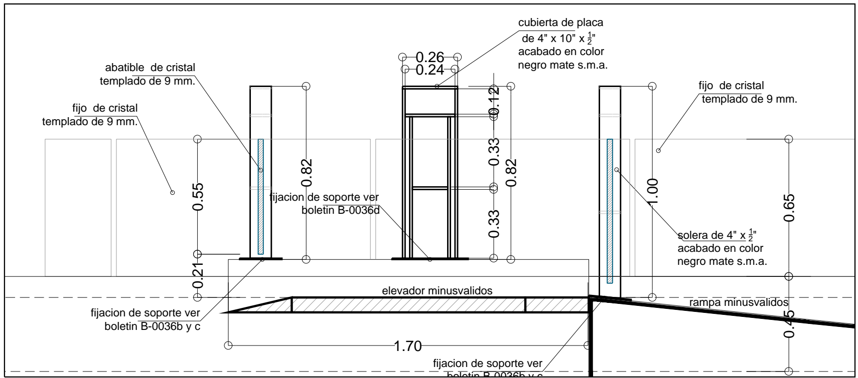
CORTE-D
