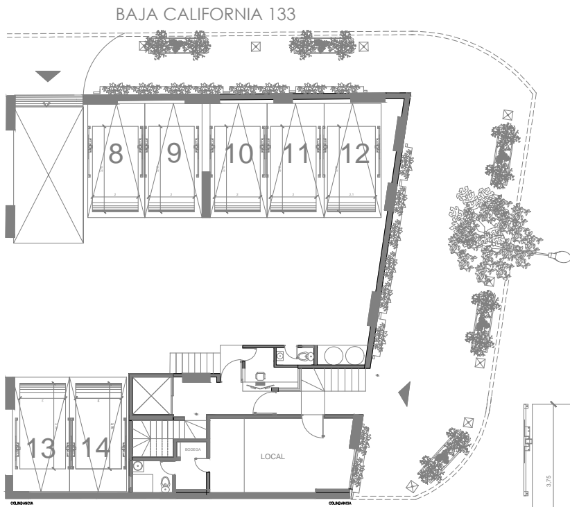
PLANTA BAJA
