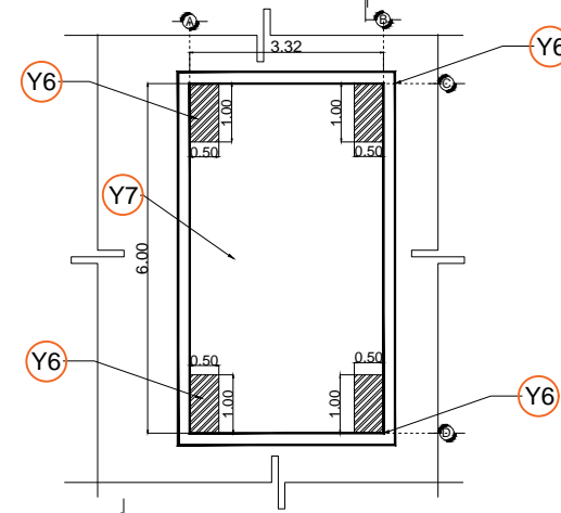
FOSO VISTA PLANTA
