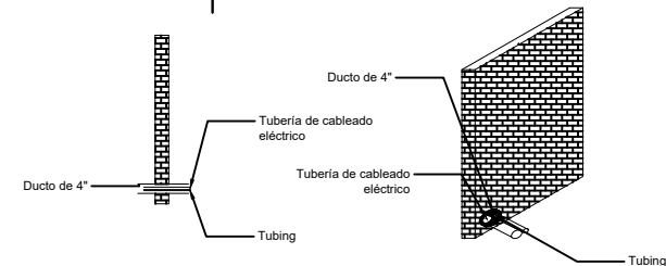
ARMADO DE FIRME PARA UNIDAD HIDRAULICA
