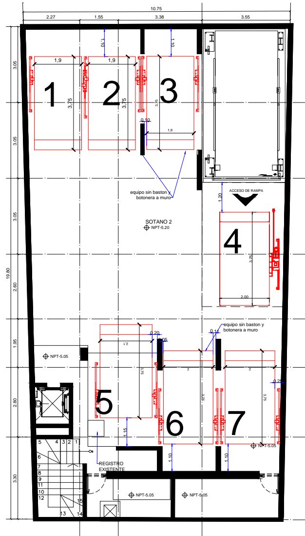
00 PLANTA SOTANO 2 PLANTA ARQUITECTONICA
