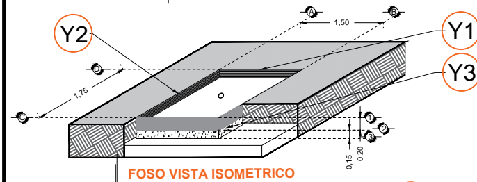
FOSO-VISTA ISOMETRICO
