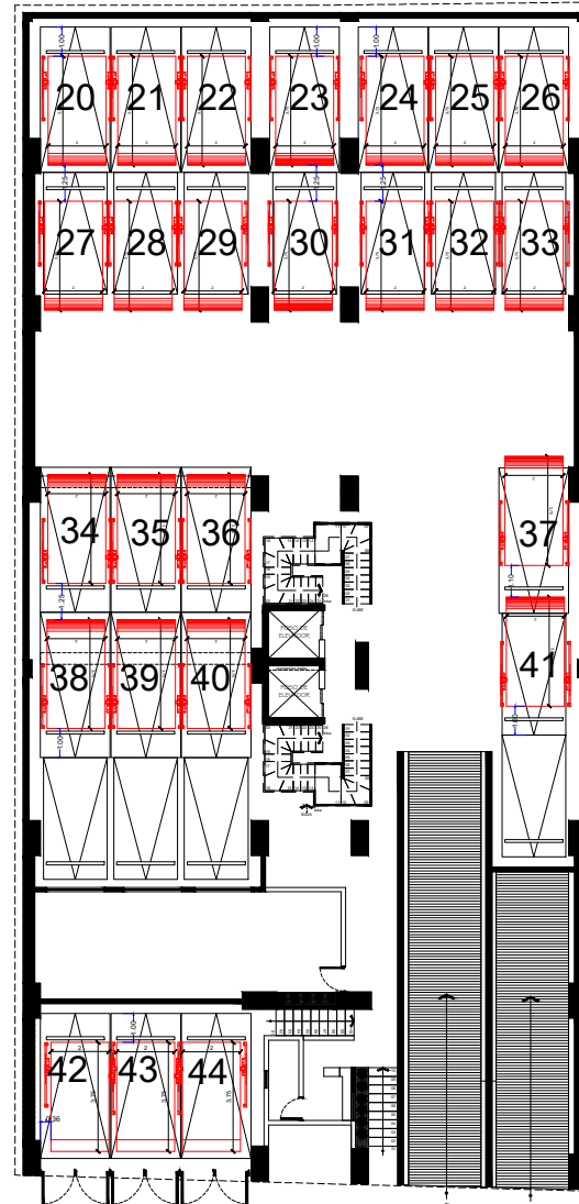
PLANTA BAJA NPT. + 1.80
