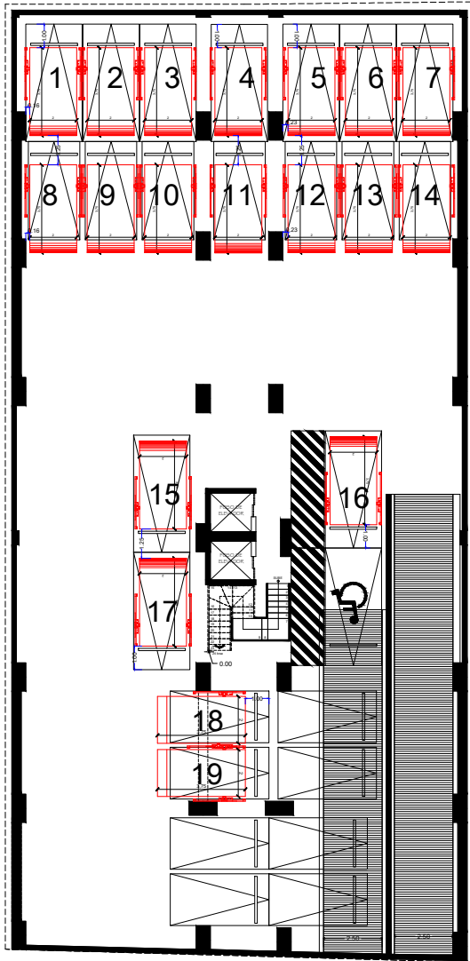
PLANTA SOTANO ESTACIONAMIENTO NPT. -2.40
