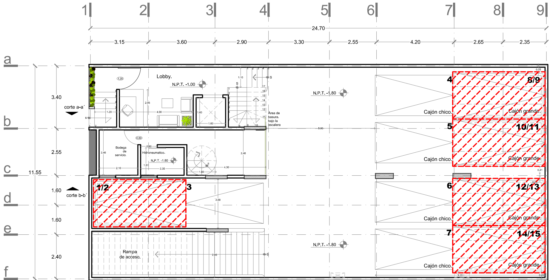
PLANTA DE SEMISOTANO N.P.T -1.80 mts.
