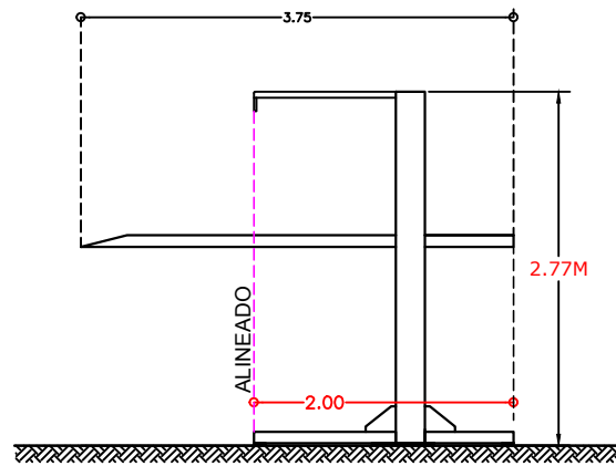
VISTA LATERAL
