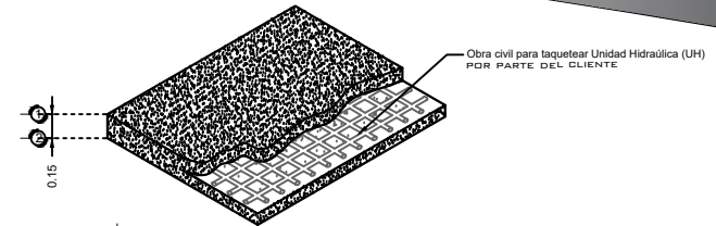
ARMADO DE FIRME PARA UNIDAD HIDRÁULICA
